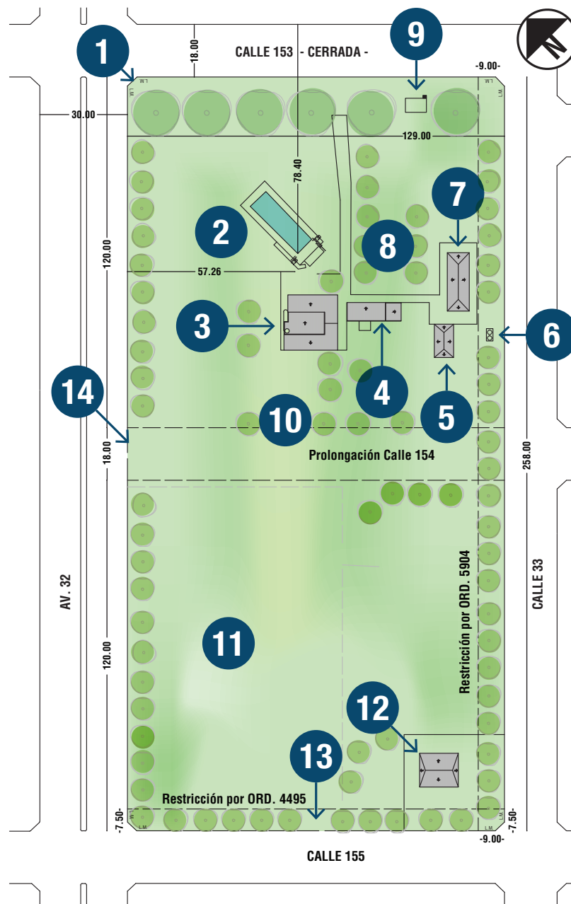
Planta del predio El Campito. Existencias y Restricciones de dominio
